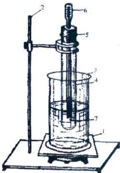
Рис. 49. Прибор для определения температуры плавления жира:
