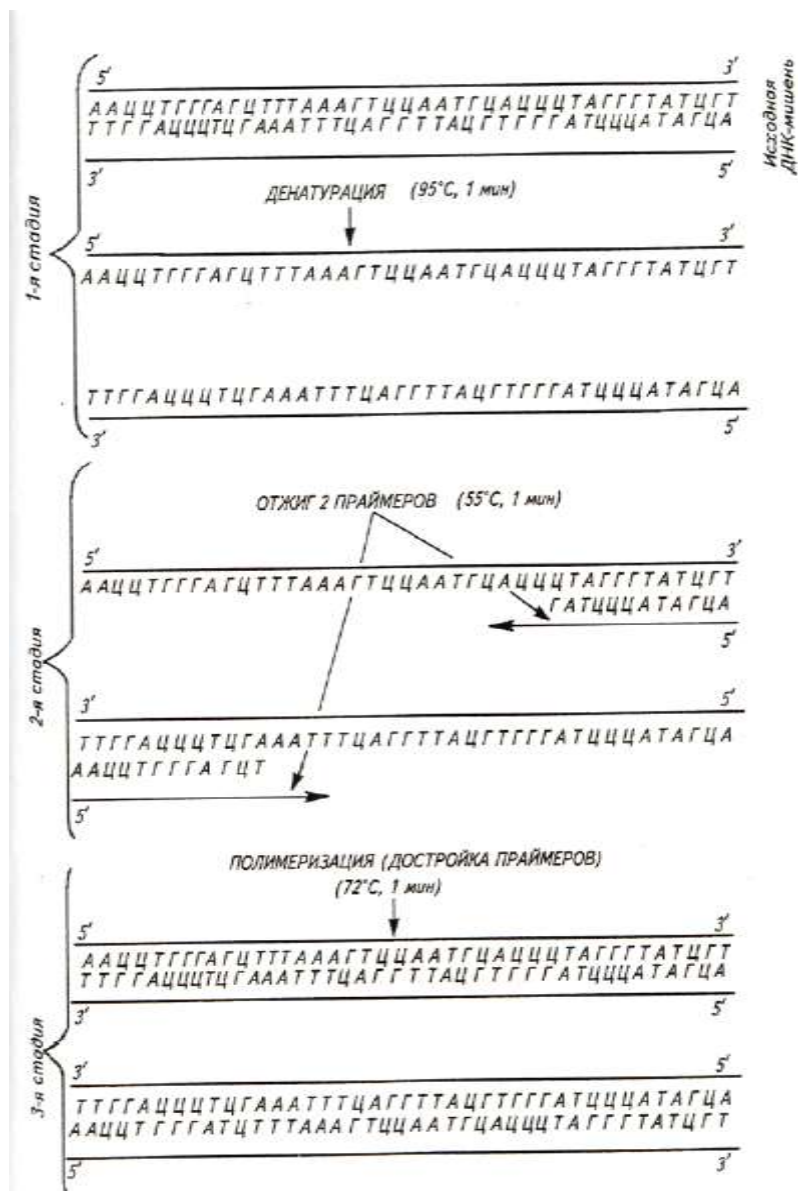
Рис. 53. Схема первого цикла ПЦР. Через два цикла будет 4 копии исходной молекулы ДНК-мишени, а через n циклов - 2^n копий.
