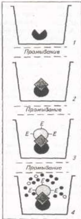
Рис. 50. Схема определения антигена методом двойных антител («сэндвич») – в твердофазном ИФА:
