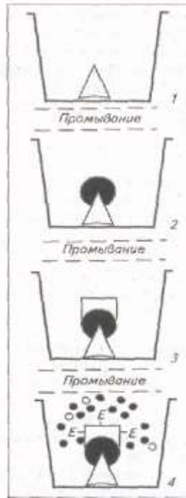
Рис. 51.Схема определения антител непрямым методом твердофазного - ИФА:
